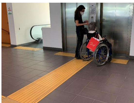
Esempio di buone prassi per la realizzazione di una efficiente segnaletica tattile a pavimento di intercettazione di un servizio, in questo caso l'ascensore, utilizzando in codice LVE.
