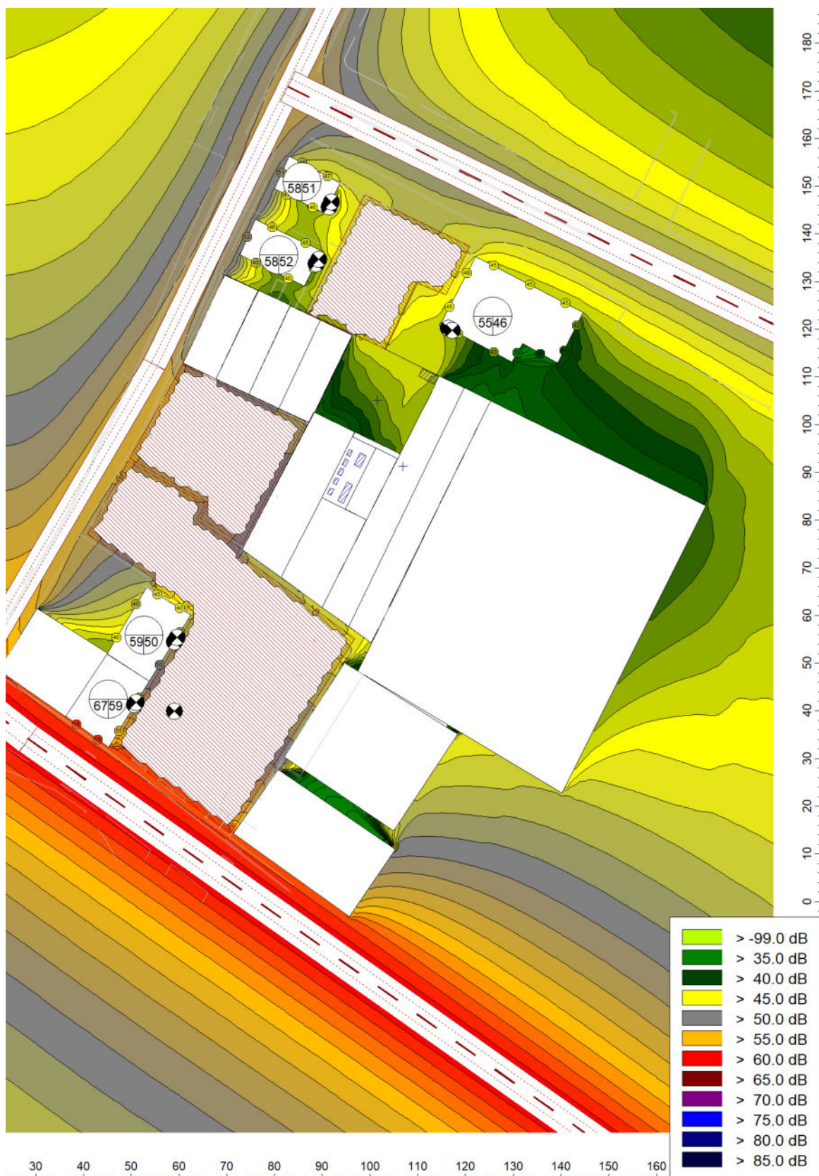
Mapa delle superfici di isolivello sonoro in periodo notturno – COMPLESSIVO, h 4,0 m
