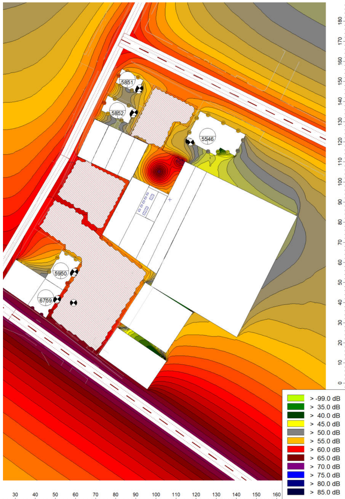
Mapa delle superfici di isolivello sonoro in periodo diurno – COMPLESSIVO, h 4,0 m
