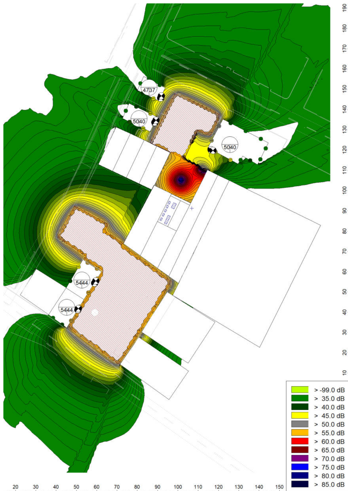
Mappe delle superfici di isolivello sonoro in periodo diurno – DIFFERENZIALE, h 1,5 m
