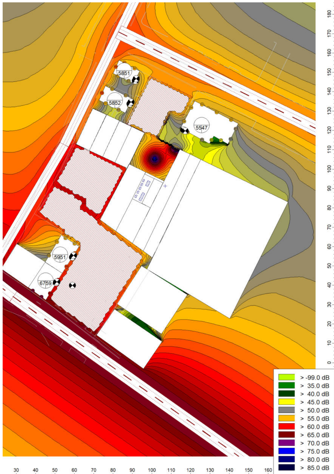
Mapa delle superfici di isolivello sonoro in periodo diurno – COMPLESSIVO, h 1,5 m
