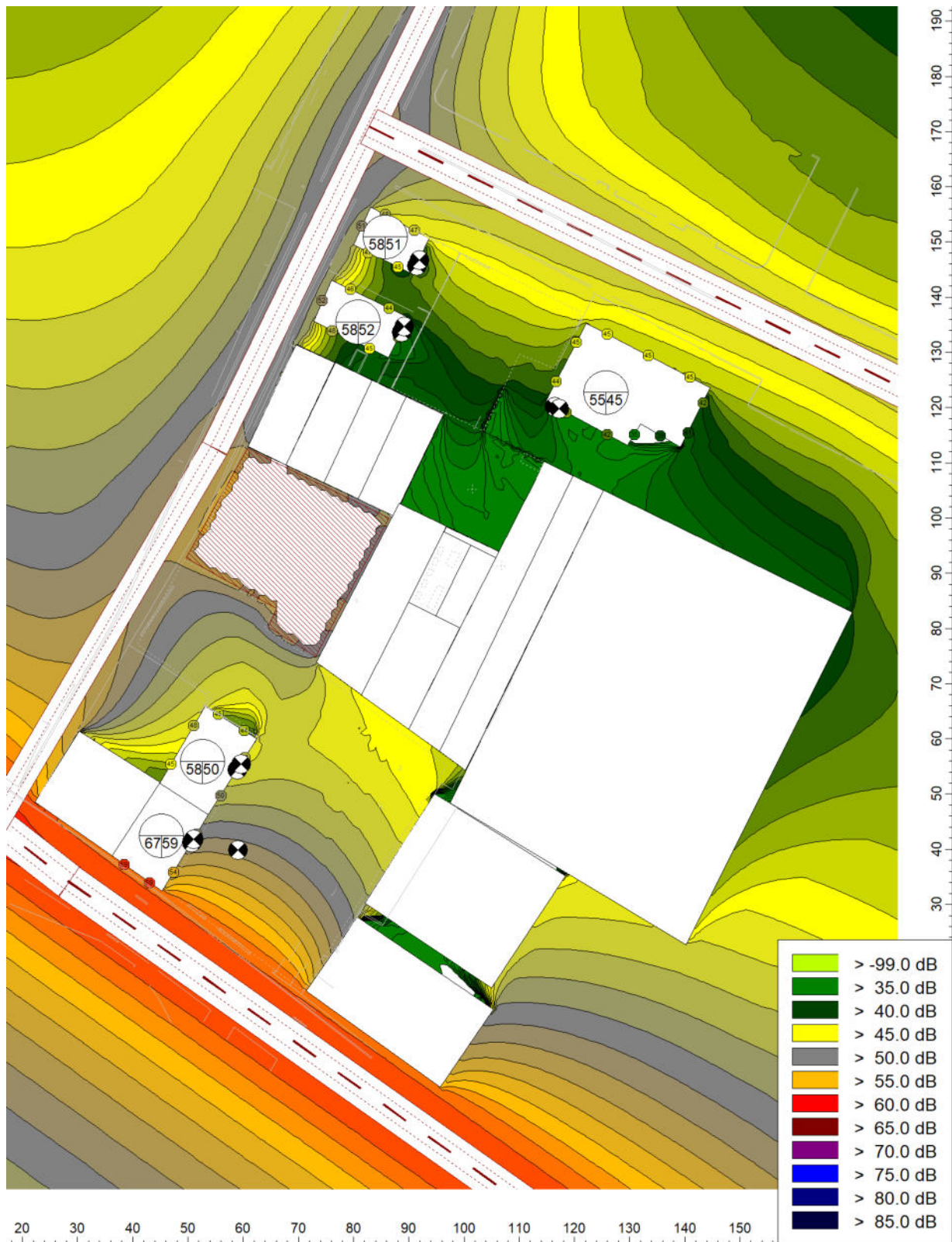
Mapa delle superfici di isolivello sonoro in periodo notturno – ASSOLUTO, h 1,5 m
