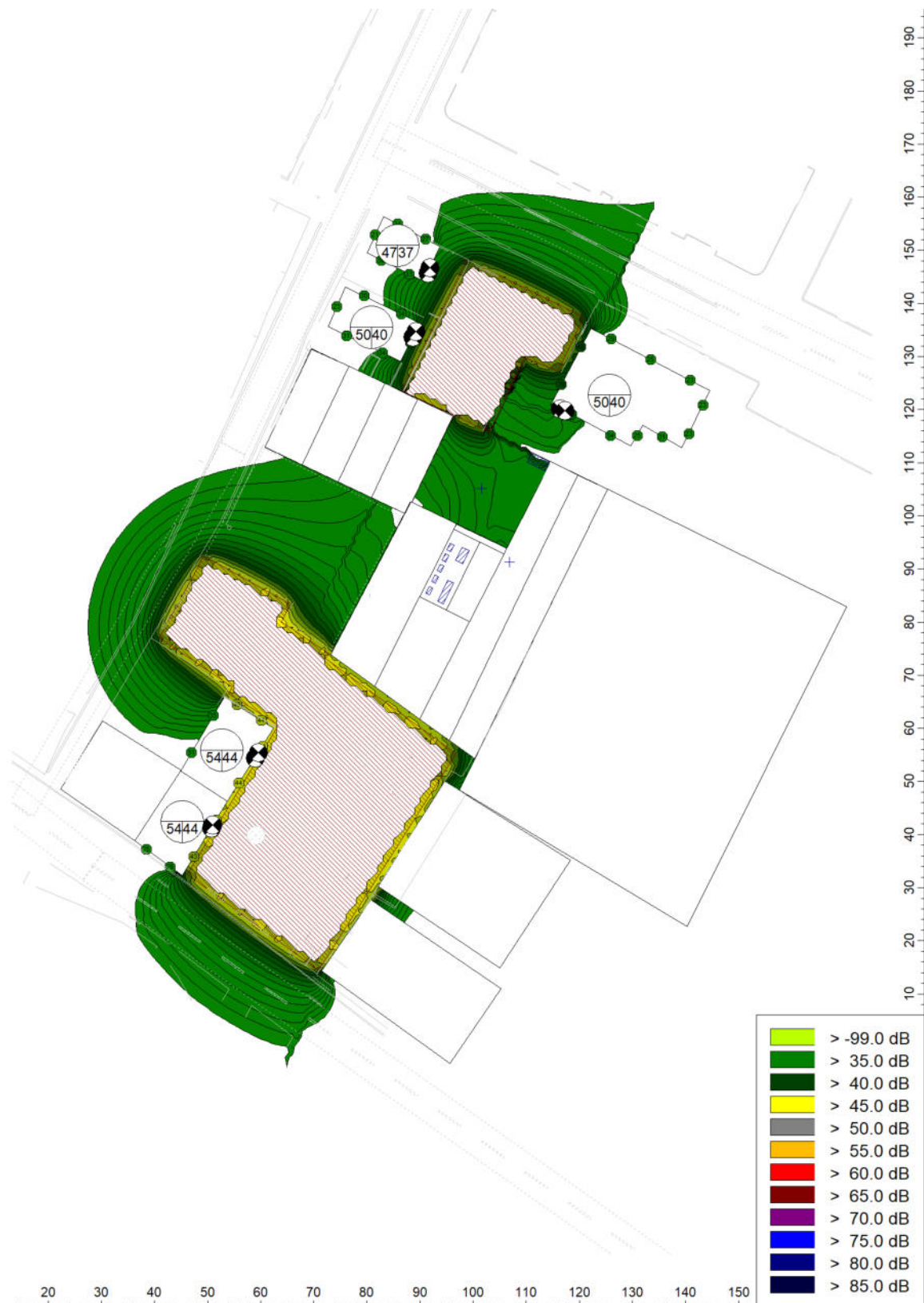
Mapa delle superfici di isolivello sonoro in periodo notturno – DIFFERENZIALE, h 1,5 m
