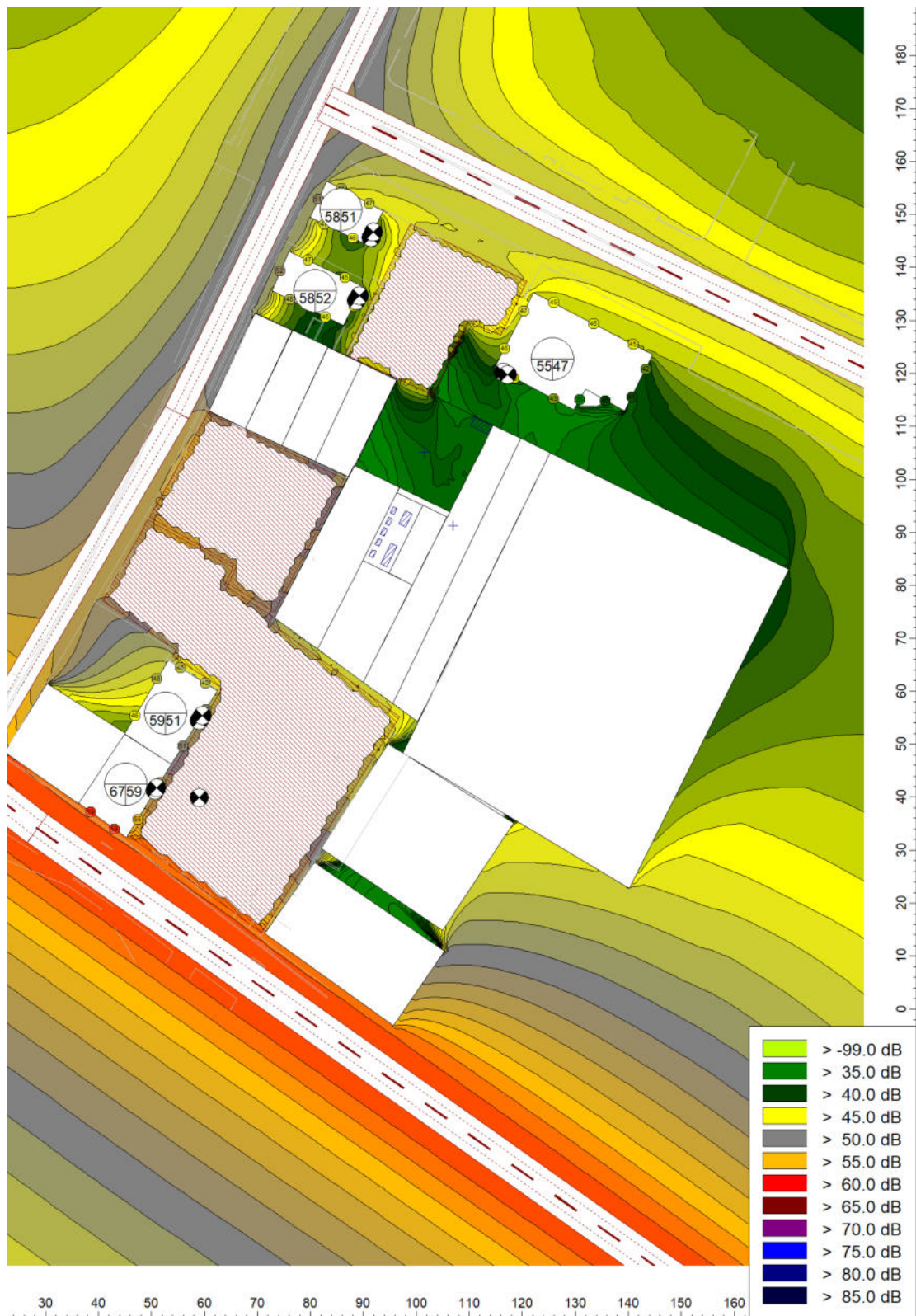
Mapa delle superfici di isolivello sonoro in periodo notturno – COMPLESSIVO, h 1,5 m
