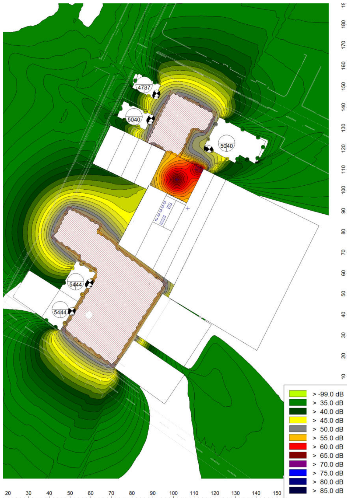
Mappa delle superfici di isolivello sonoro in periodo diurno – DIFFERENZIALE, h 4,0 m
