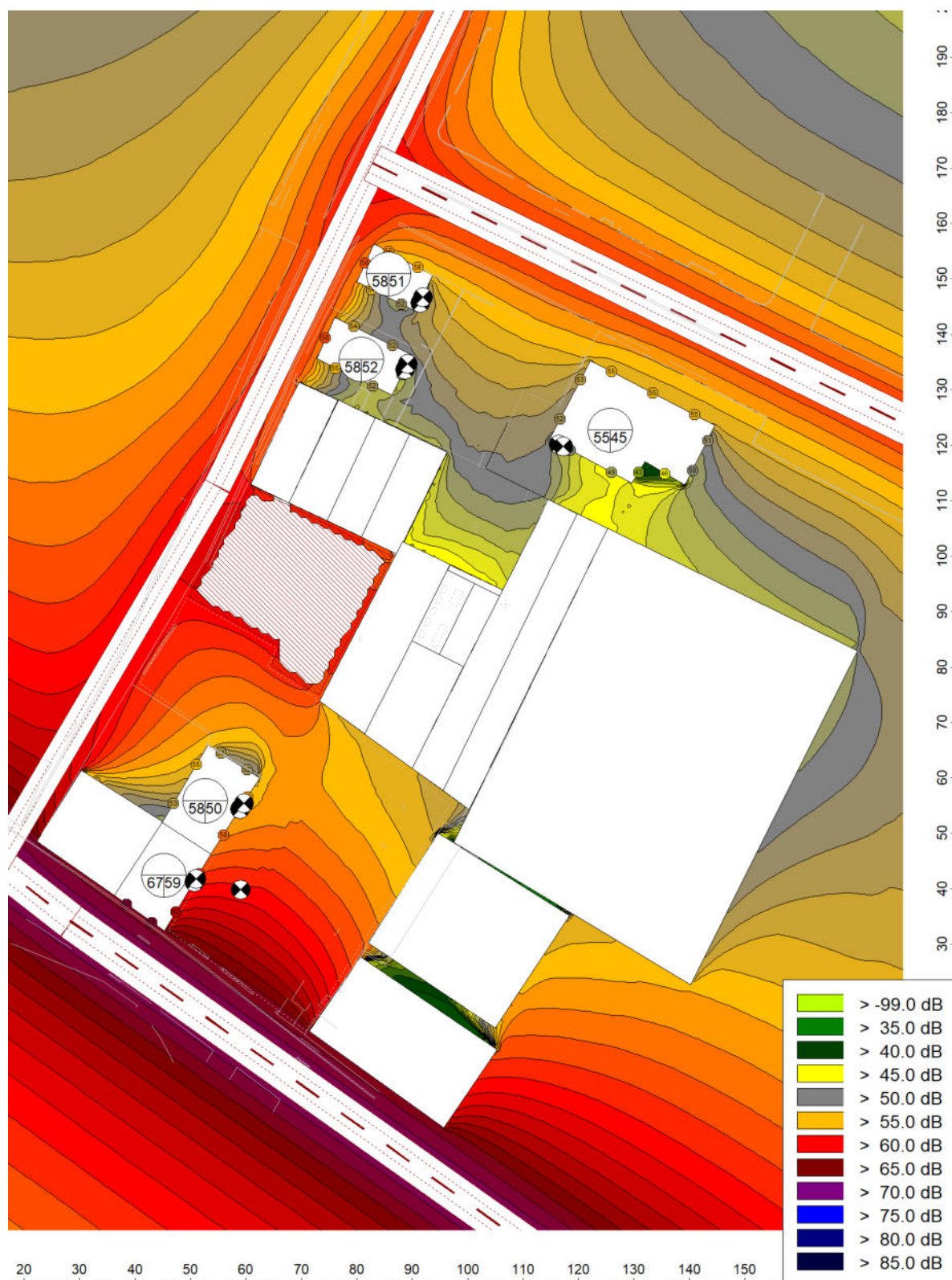
Mapa delle superfici di isolivello sonoro in periodo diurno – ASSOLUTO, h 4,0 m
