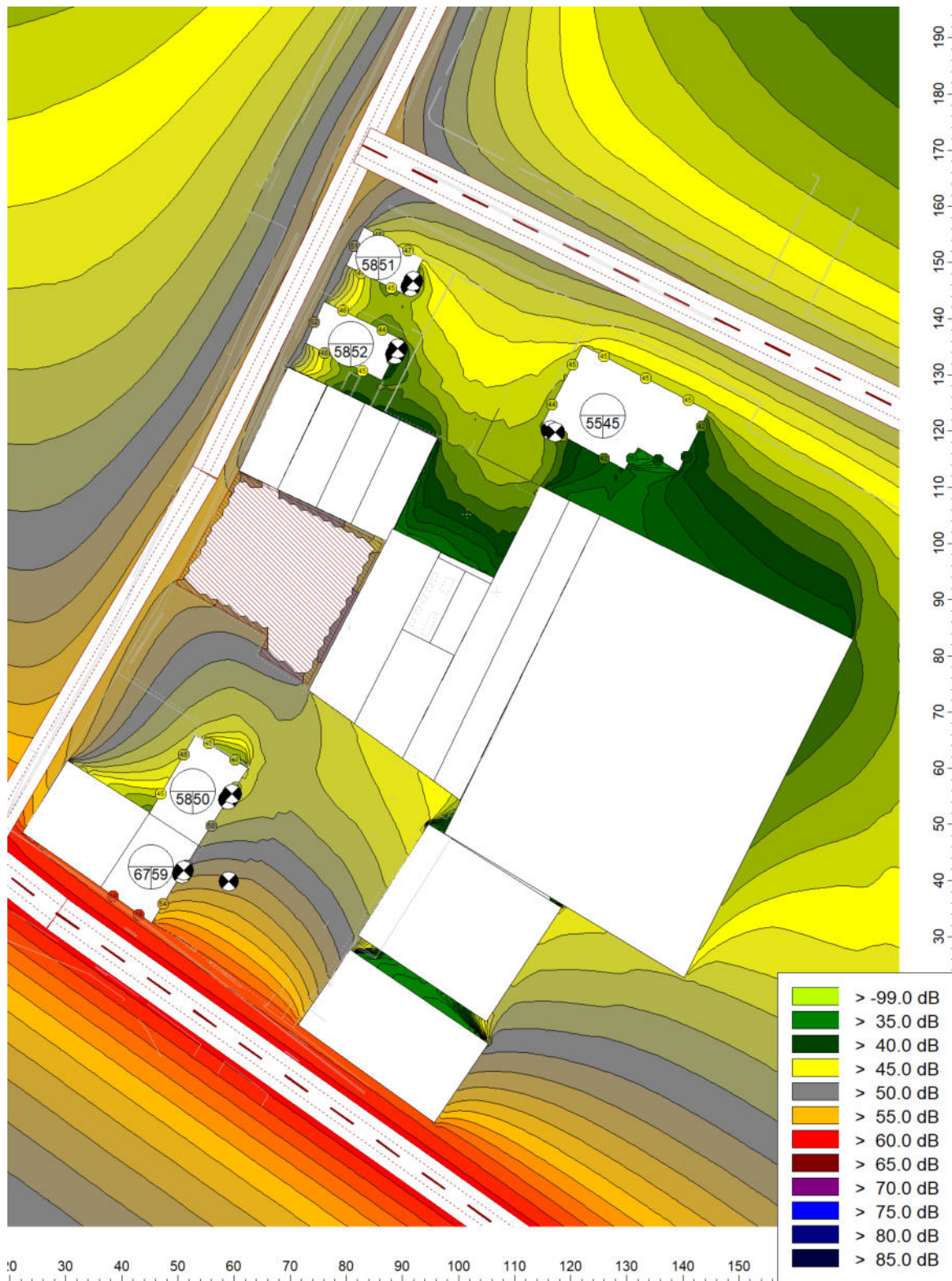
Mapa delle superfici di isolivello sonoro in periodo notturmo – ASSOLUTO, h 4,0 m
