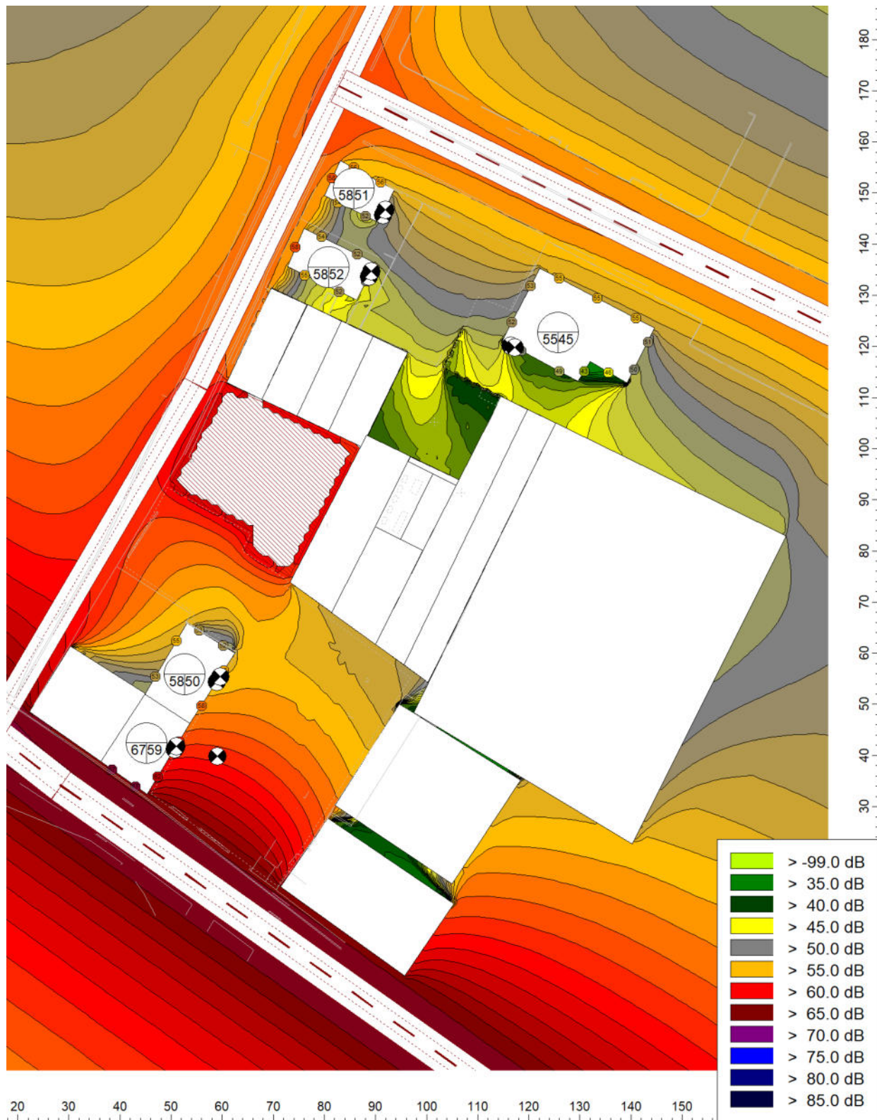
Mapa delle superfici di isolivello sonoro in periodo diurno – ASSOLUTO, h 1,5 m
