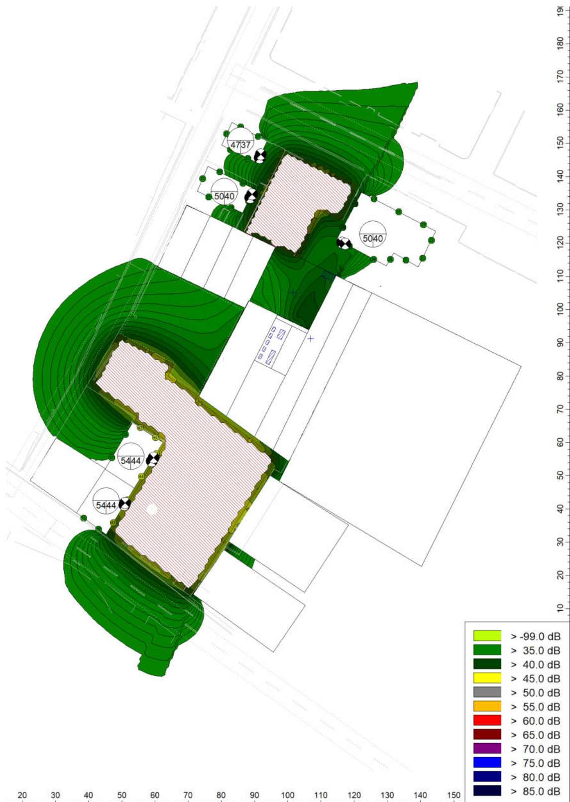
Mappa delle superfici di isolivello sonoro in periodo notturno – DIFFERENZIALE, h 4,0 m
