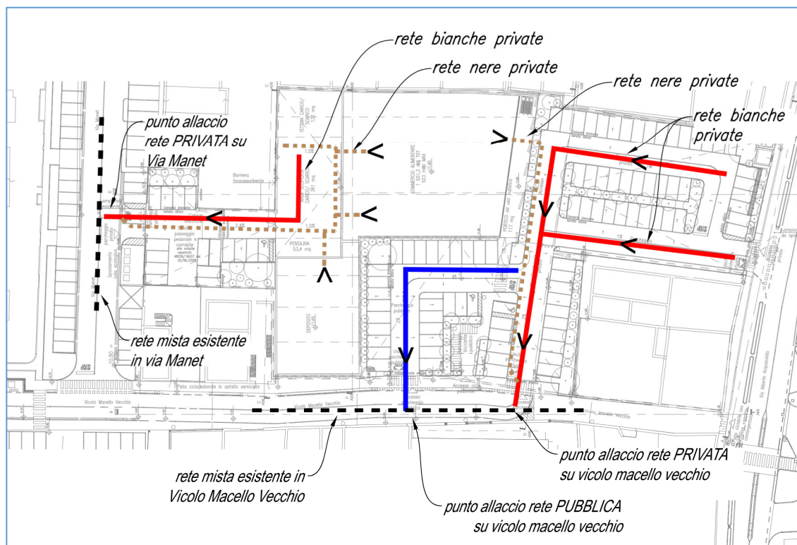
- schema fognario e allacci -
