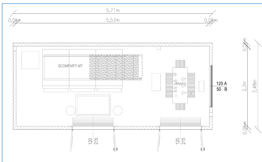
- dimensioni cabina -
