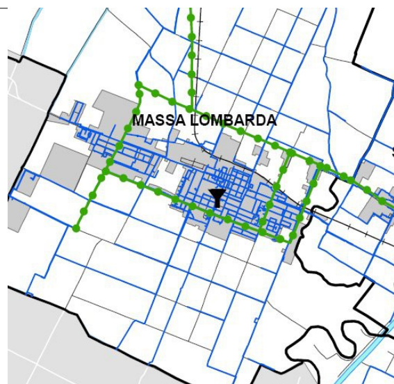
Tav.QC.7 (ST8) Rete distribuzione idrica
